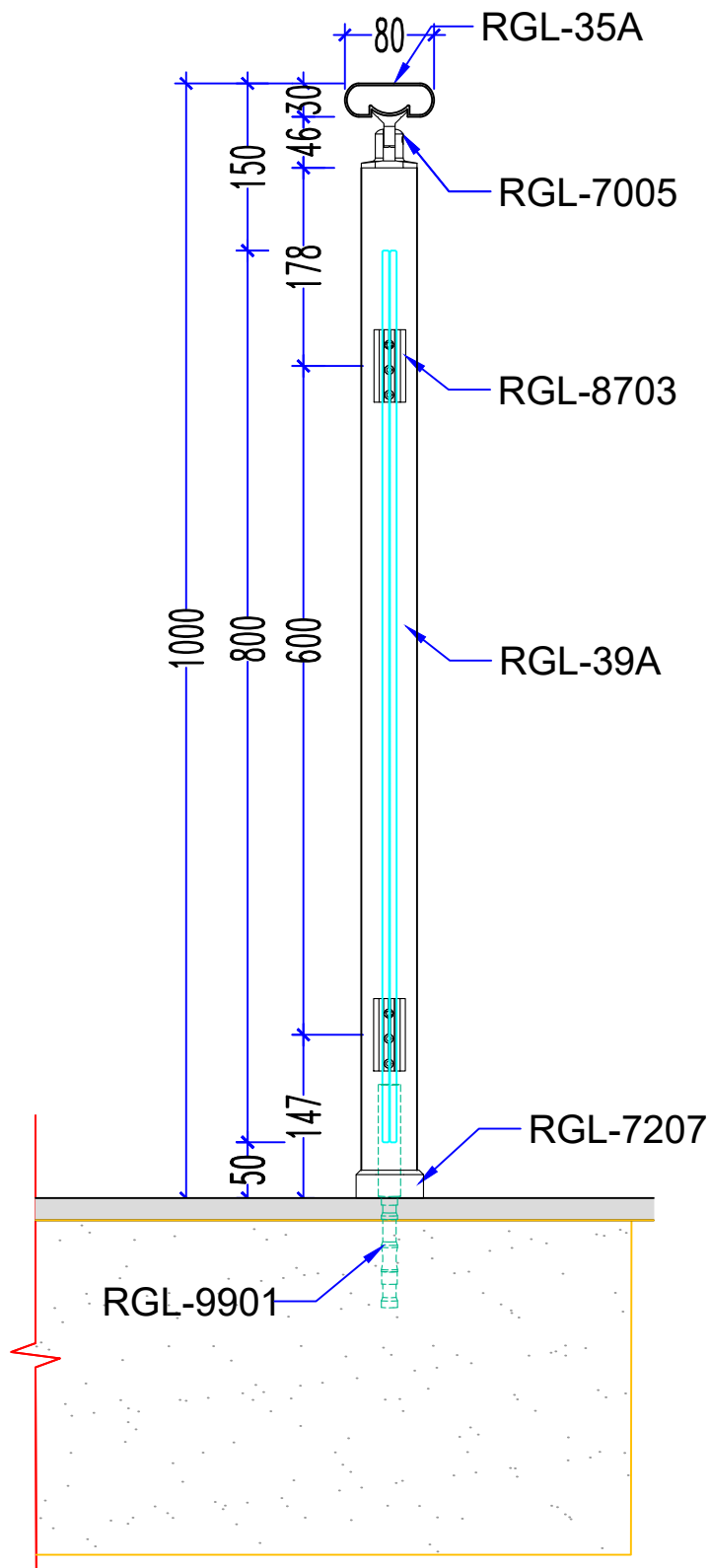
A-A SECTION
